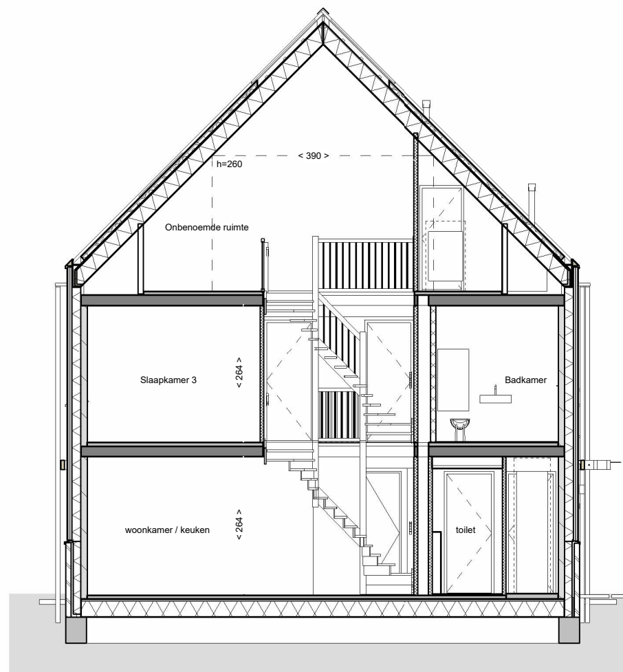
doorsnede
