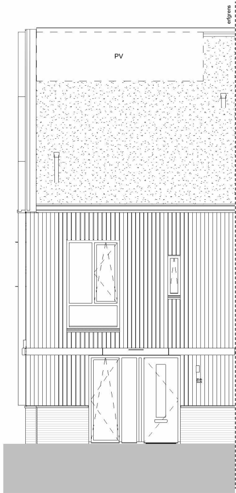
voorgevel
